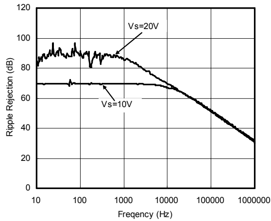
PSRR
