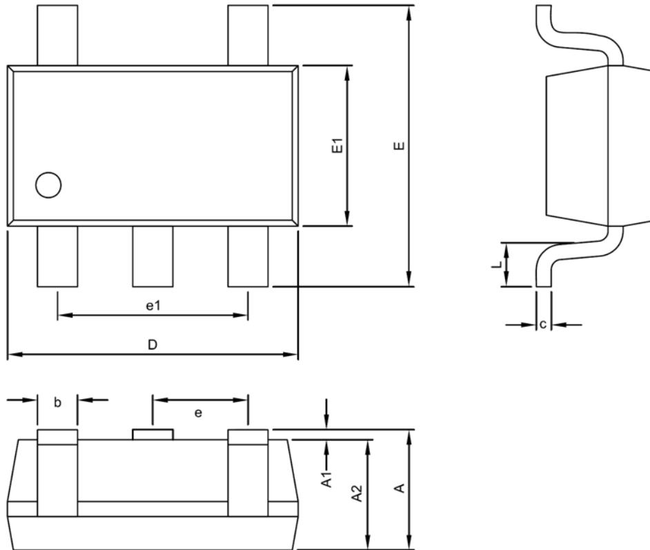
SOT-23-5 Package
