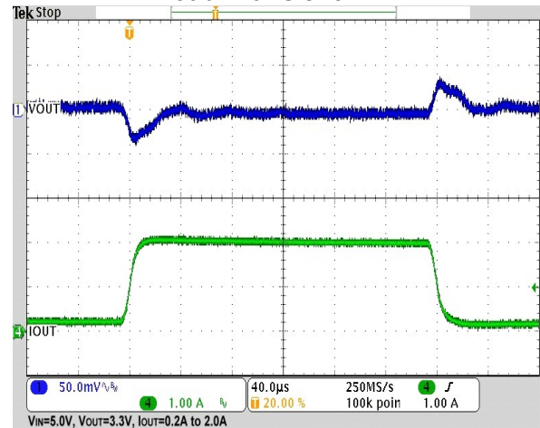
Load Transient-CH4
