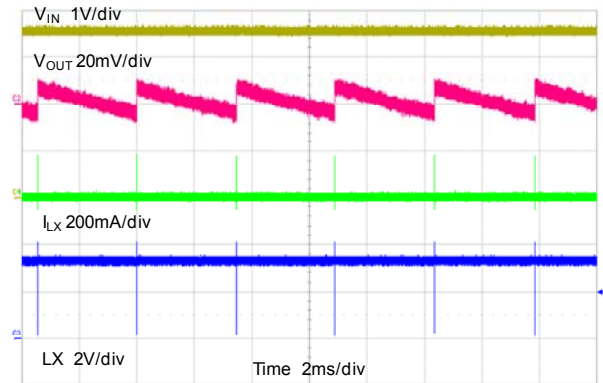
V_{IN}=3.6V , V_{OUT}=3.3V , No Load
