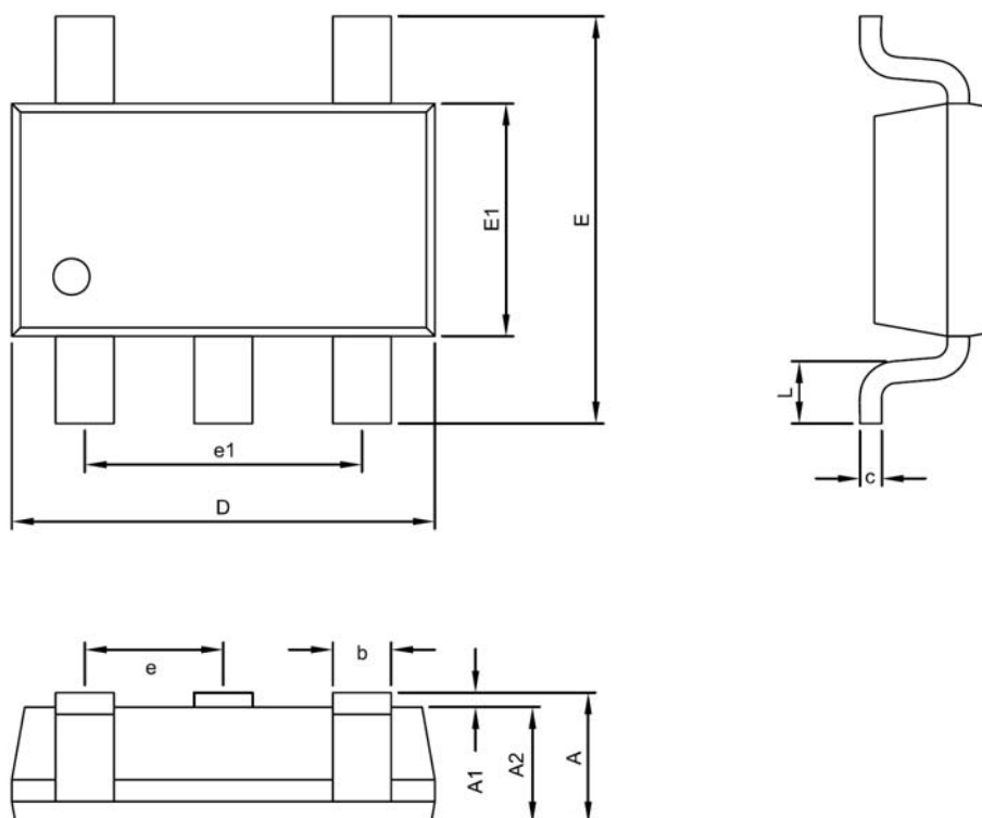
TSOT-23-5 Package
