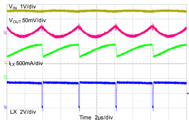
V_{IN}=3.6V , V_{OUT}=3.3V , I_{OUT}=1A
