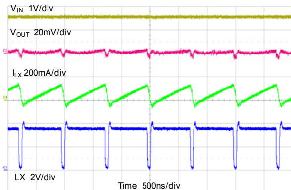
V_{IN}=3.6V , V_{OUT}=3.3V , I_{OUT}=50mA
