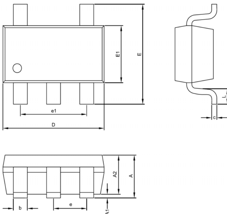
SOT-23-5 Package
