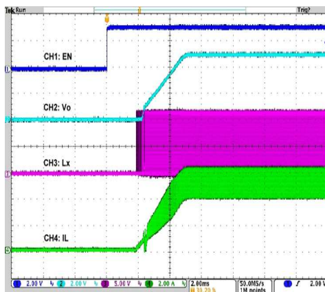
EN ON
