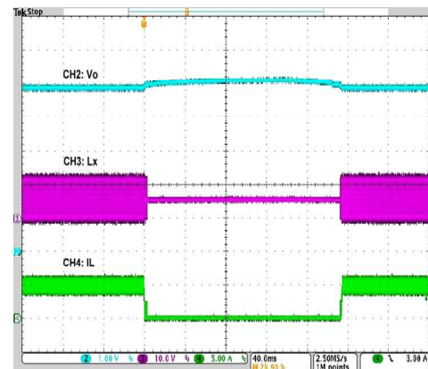
OVP
