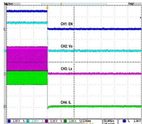
EN OFF
