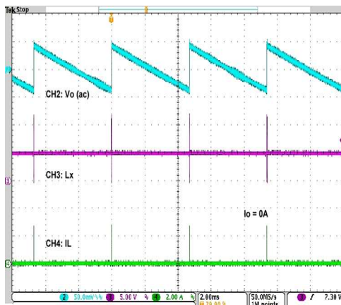
Ripple
