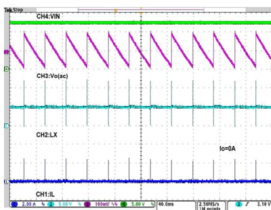
Ripple
