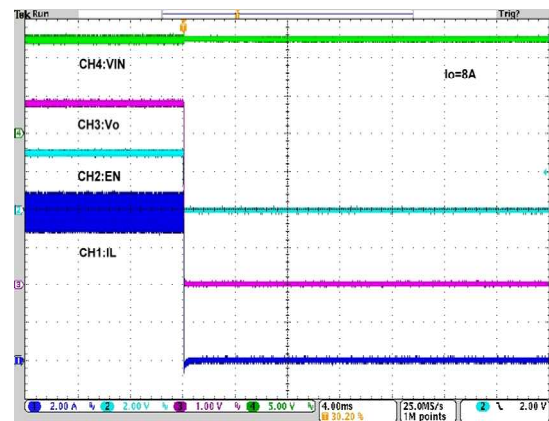
EN OFF
