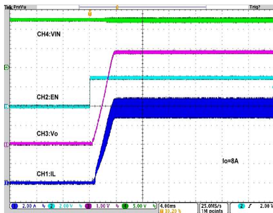
EN ON
