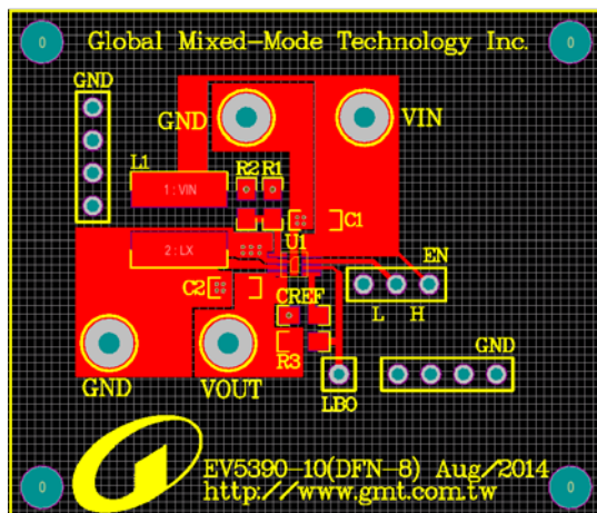
Top Layer
