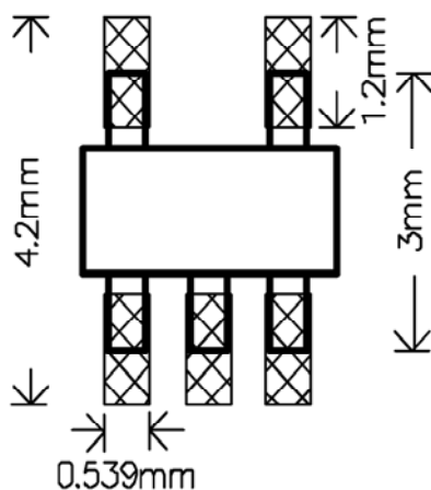
SOT-23-5/TSOT-23-5
