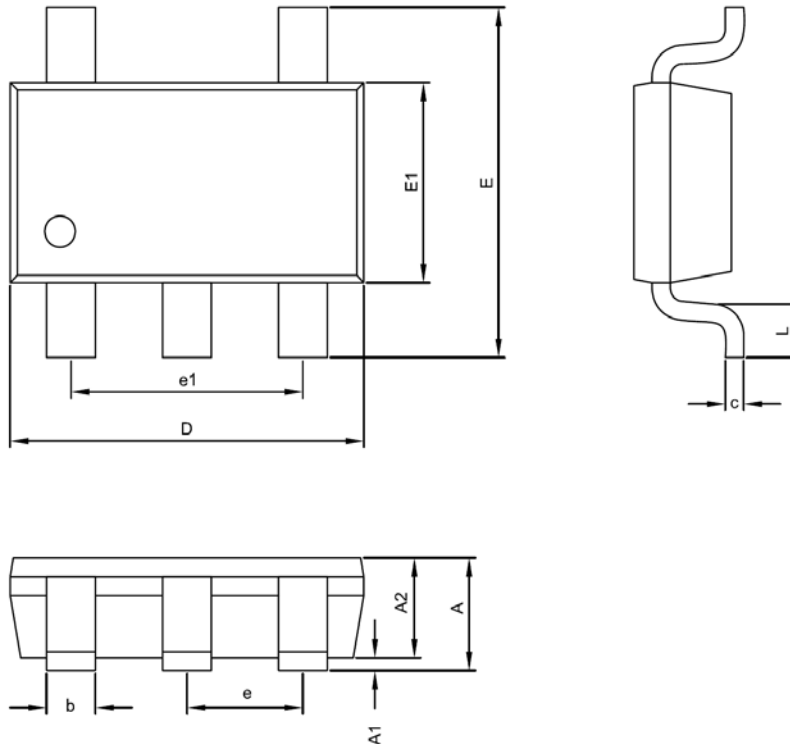
TSOT-23-5 Package
