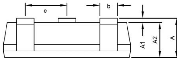
TSOT-23-5 Package
