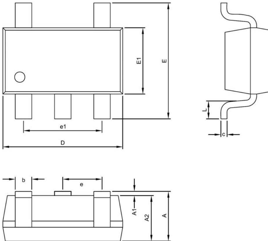
SOT-23-5 Package
