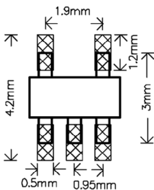
SOT-23-5/TSOT-23-5
