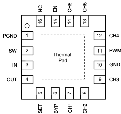
G5966L TQFN3X3-16
