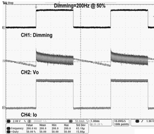
Dimming (duty & io)
