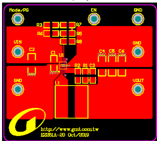
Top Layer
