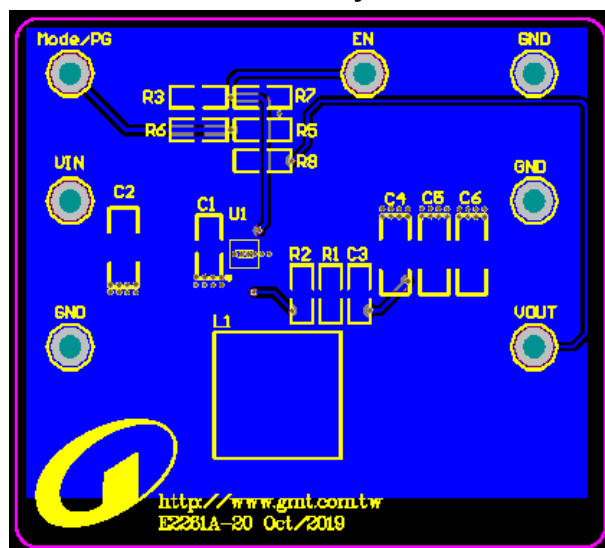
Bottom Layer
