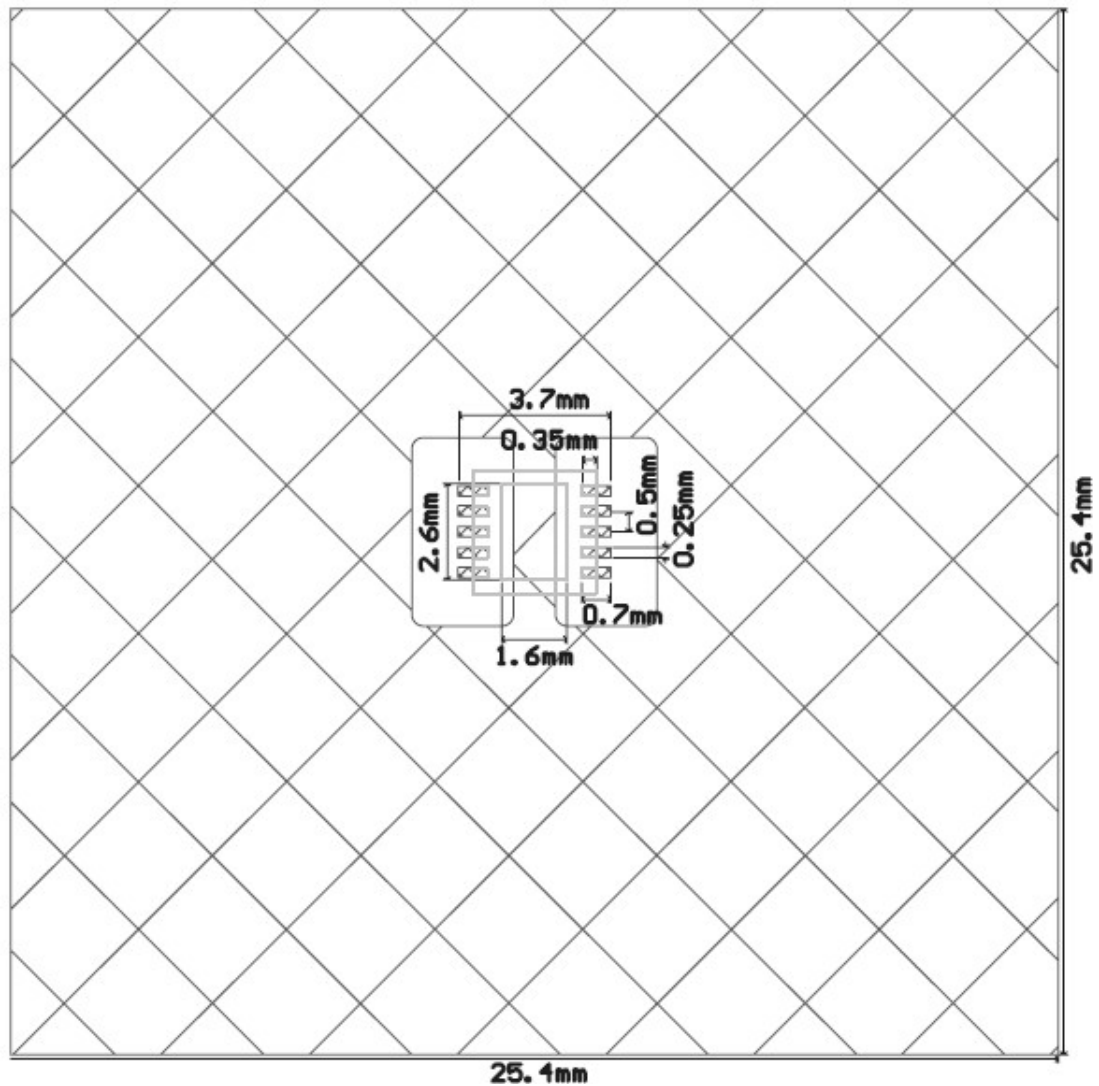
TDFN3X3-10
