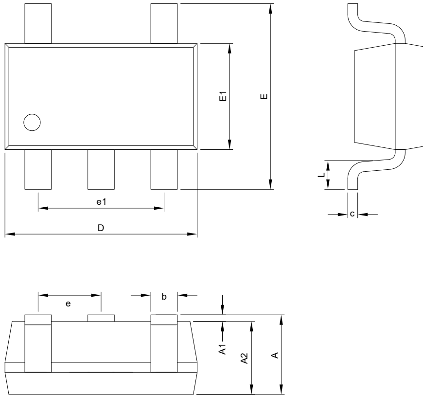
SOT-23-5 Package
