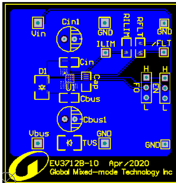
Bottom Layer
