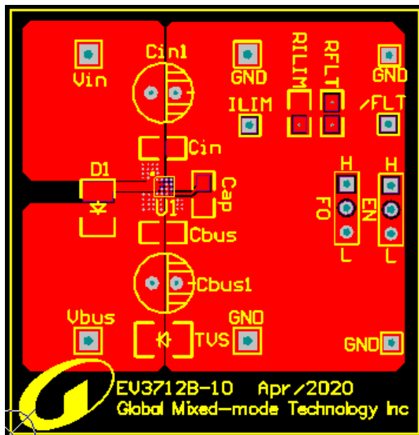
Top Layer
