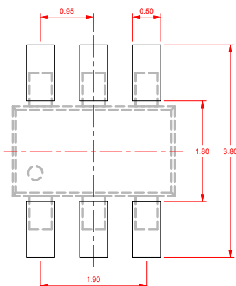
SOT-23-6/TSOT-23-6
