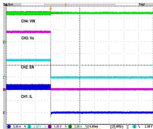
EN OFF
