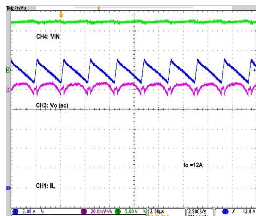
Ripple
