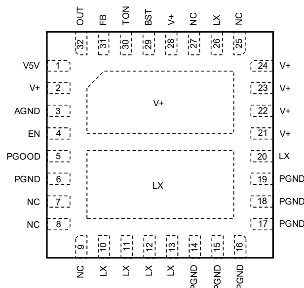
G5329A QFN4X4-32
