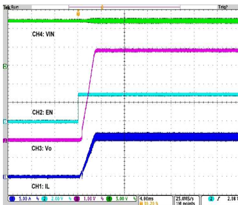
EN ON
