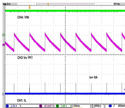
Ripple
