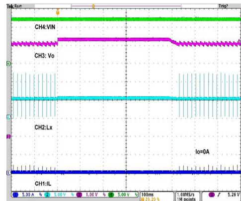
OVP
