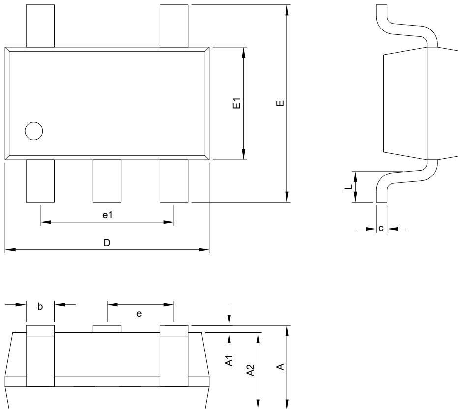
SOT-23-5 Package
