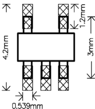
SOT-23-5/TSOT-23-5
