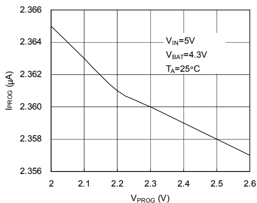
I_PROG(μA) vs V_PROG(V)
