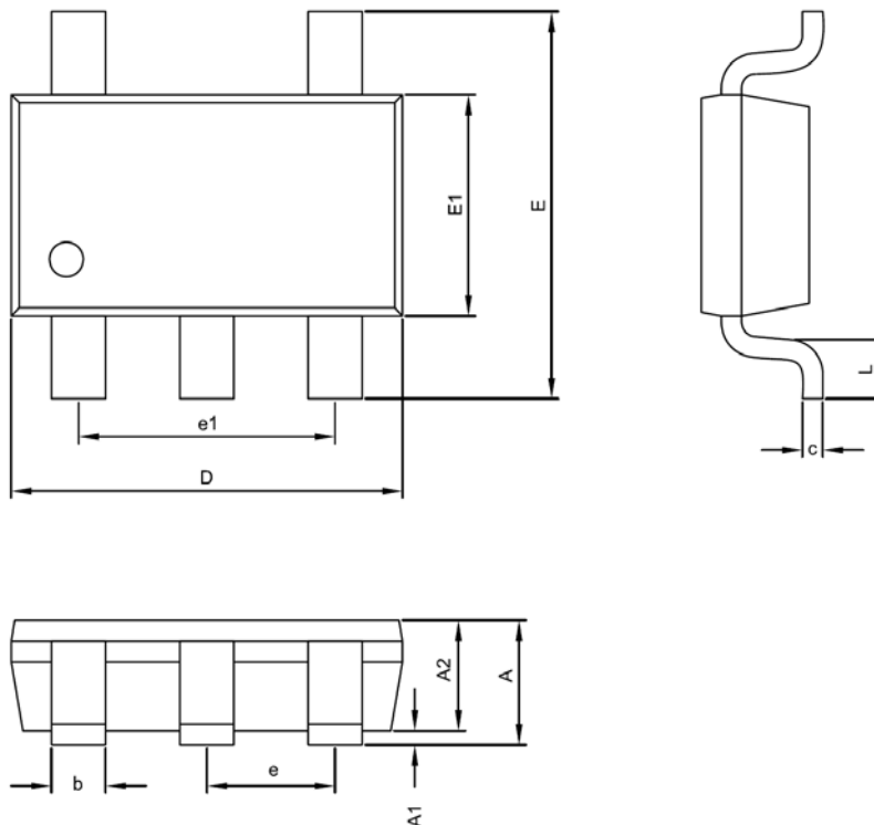
SOT-23-5 Package
