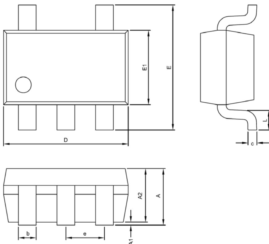
SC-70-5(SOT-353) (TA) Package
