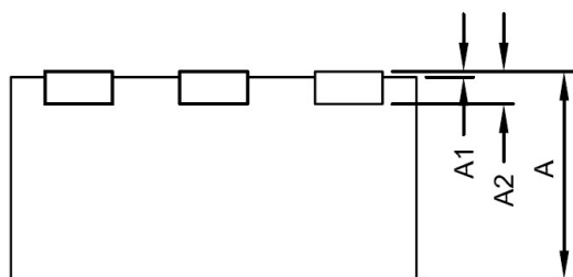
AQFN1.5X1.5-8 Package
