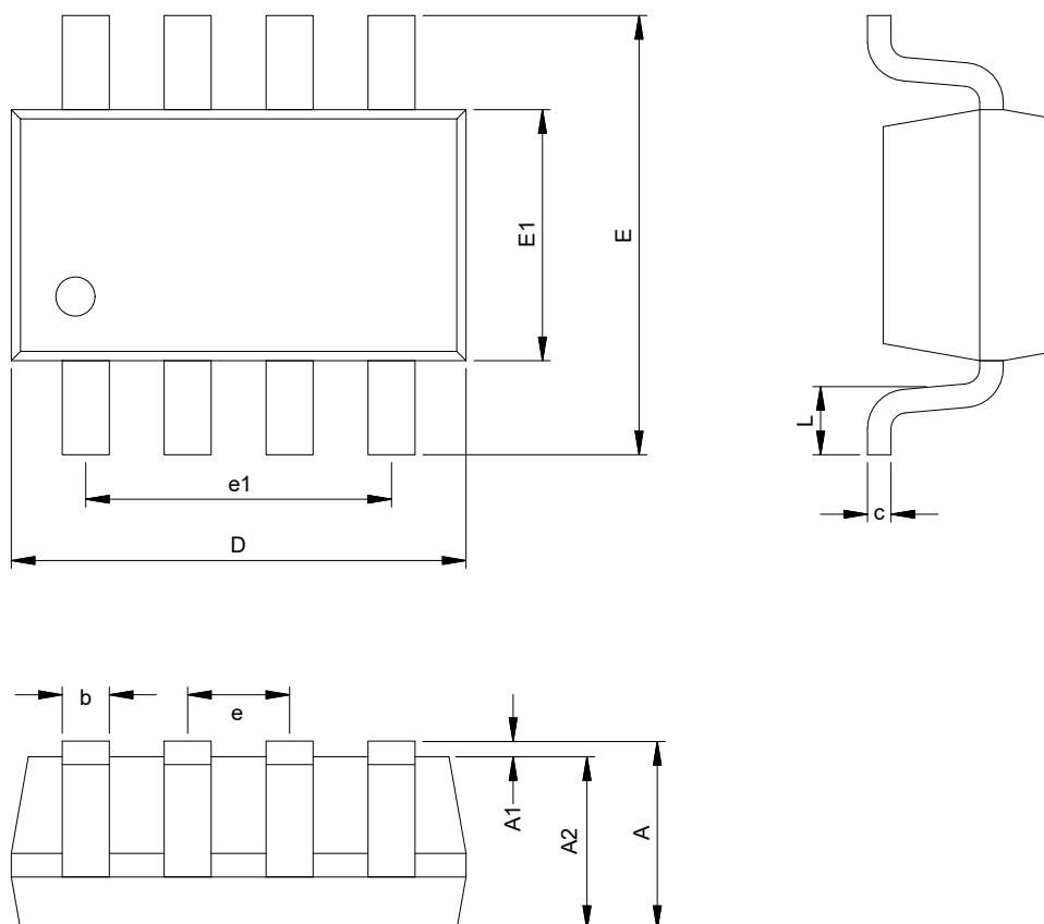
SOT-23-8 Package
